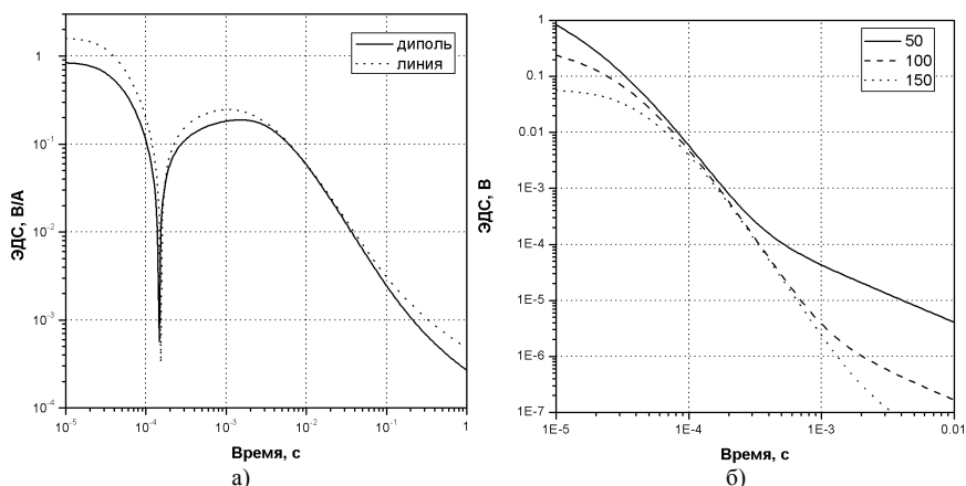
Рис. 1. Численное моделирование откликов для среды с погружённым поларизующимся слоем: а) сопоставление дипольного приближения и установки конечных размеров; б) отклики магнитовязкой среды для установок с эквивалентным моментом и разными размерами генераторных петель (шифр кривых - длина стороны генераторной петли, м).
