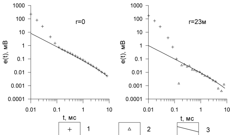
Рис. 3. Результат автоматической совместной инверсии многоразностного зондирования МПП. 1, 2 – измеренная ЭДС: 1 – положительной, 2 – отрицательной полярности; 3 – синтетическая ЭДС.
