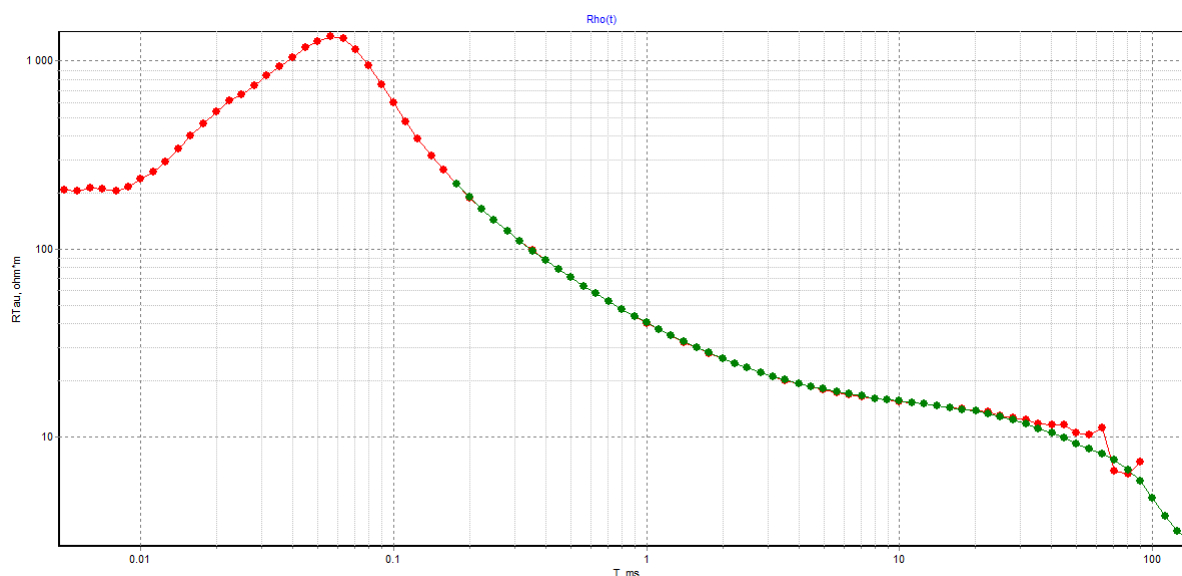
Рис. 2. Кривые кажущегося сопротивления, полученные при измерении одновитковой петлей 50×50 метров на пикете ЗСБ 11: красная – 2019 г., зеленая – 2008г.
