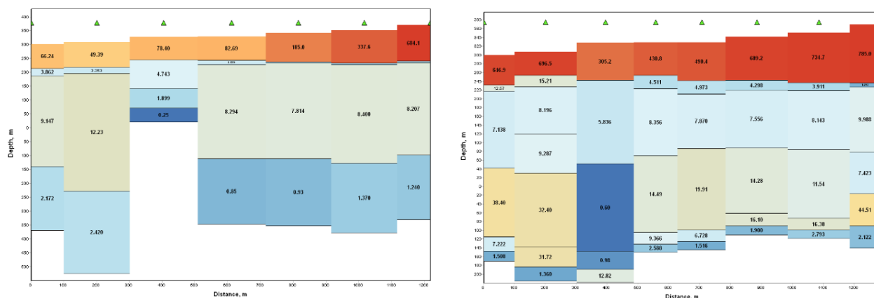
Рис. 3. Геоэлектрические разрезы на участке «Кристалл» (профиль запад–восток): слева – 2008 год, справа – 2008/2019 гг.
