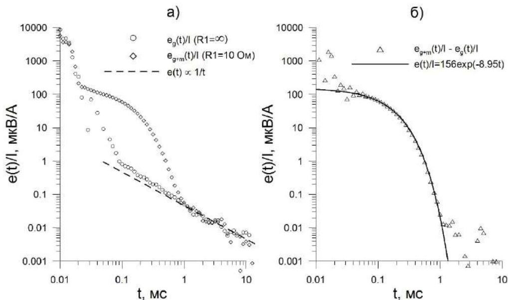
Рис. 2. Результаты тестирования для установки, расположенной в центре ( X=0 ) петли-модели (см. рис. 1, а):
