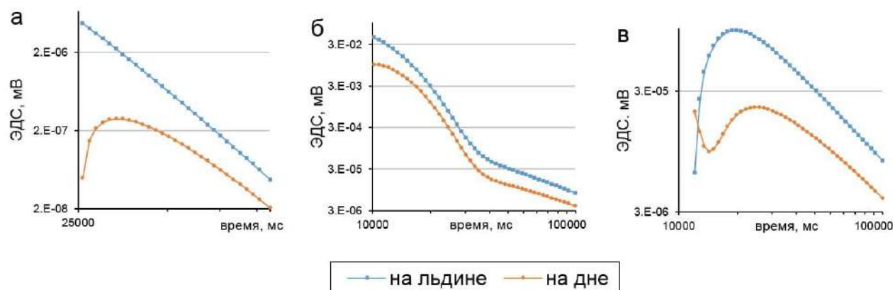
Рис. 8. Сравнение кривых становления на дне и на поверхности в точке X = 8\,000 , Y = 5\,000 : а) кривые dB_z/dt ; б) кривые E_r суммарное; в) кривые E_r аномальное
