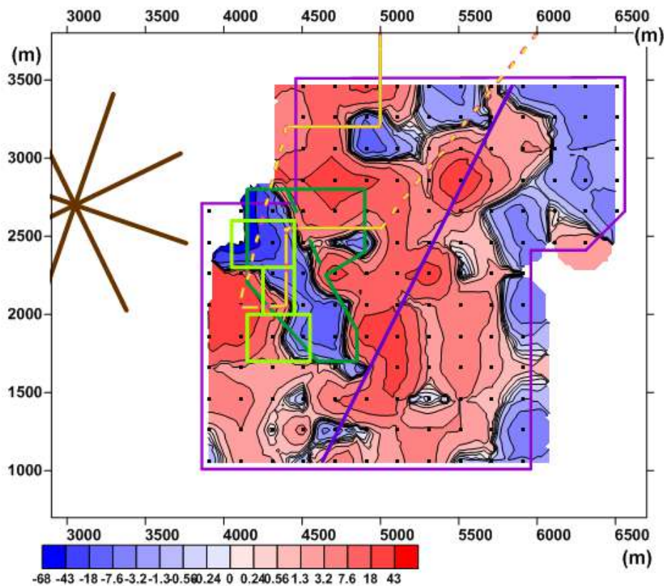
Рис. 2. Сигналы компоненты \partial B_z / \partial t работ ЗВТ, время 0,79 мс, Восточный Казахстан
