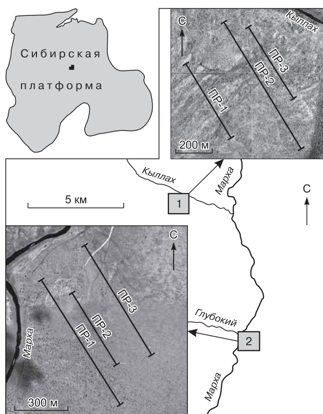
Рис. 1. Схемы геофизических профилей на участках Файнштейновский (1) и Байтахский (2), располагающихся в пределах Алаakit-Мархинского кимберлитового поля (Западная Якутия).
