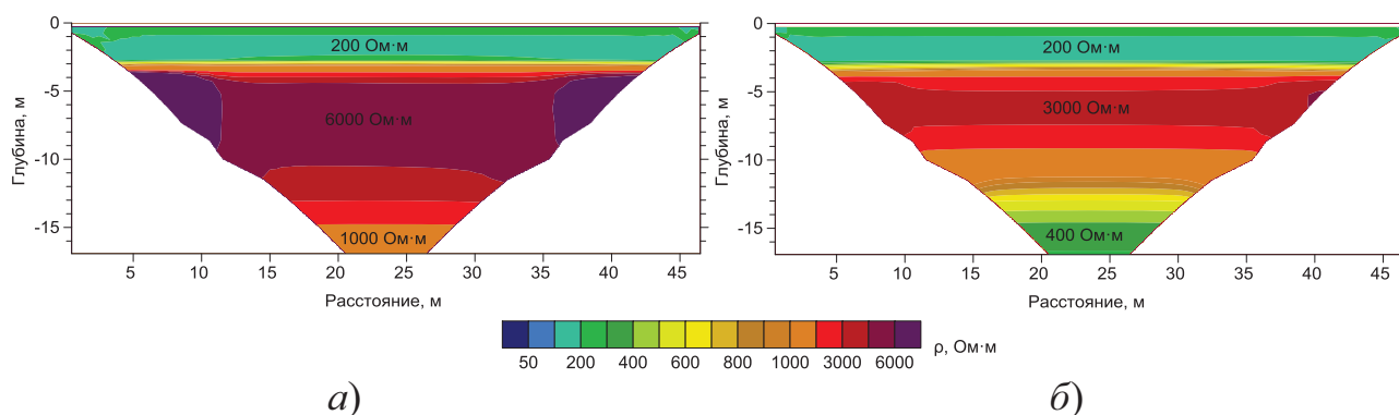
Рис. 3. Геоэлектрические разрезы по профилю внутри пещеры:
