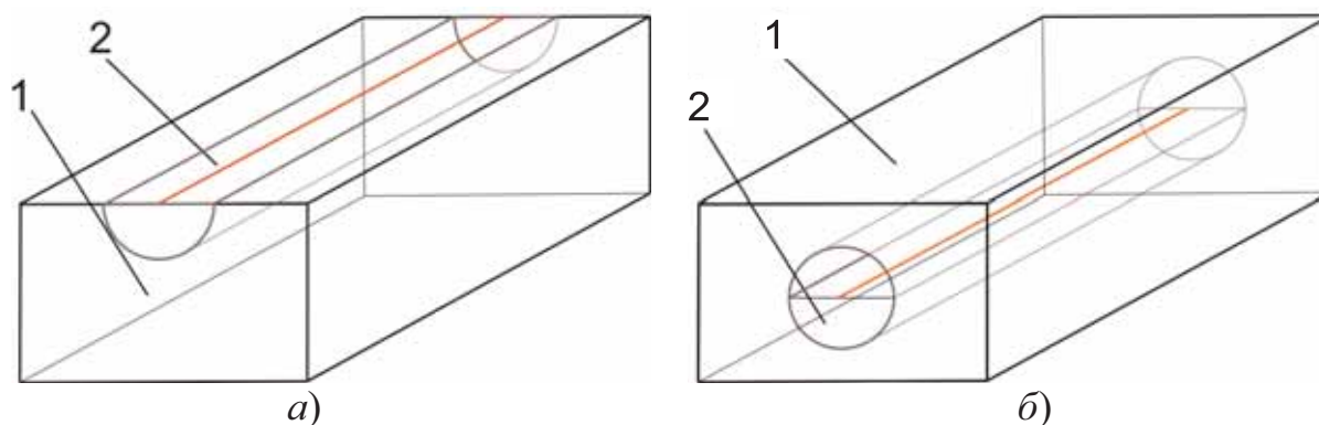
Рис. 2. Модели пещеры:
