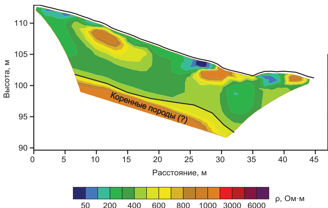
Рис. 1. Геоэлектрический разрез по профилю внутри пещеры
