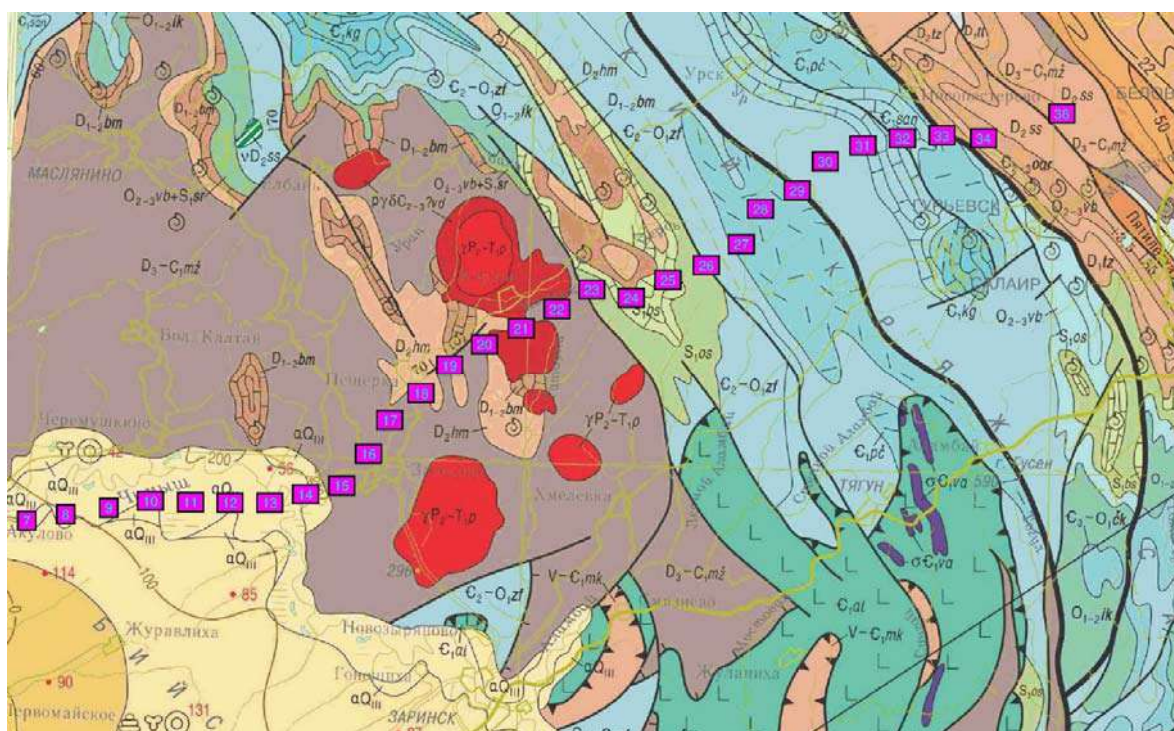
Рис. 1. Фрагмент геологической карты со схемой расположения пунктов МТЗ
