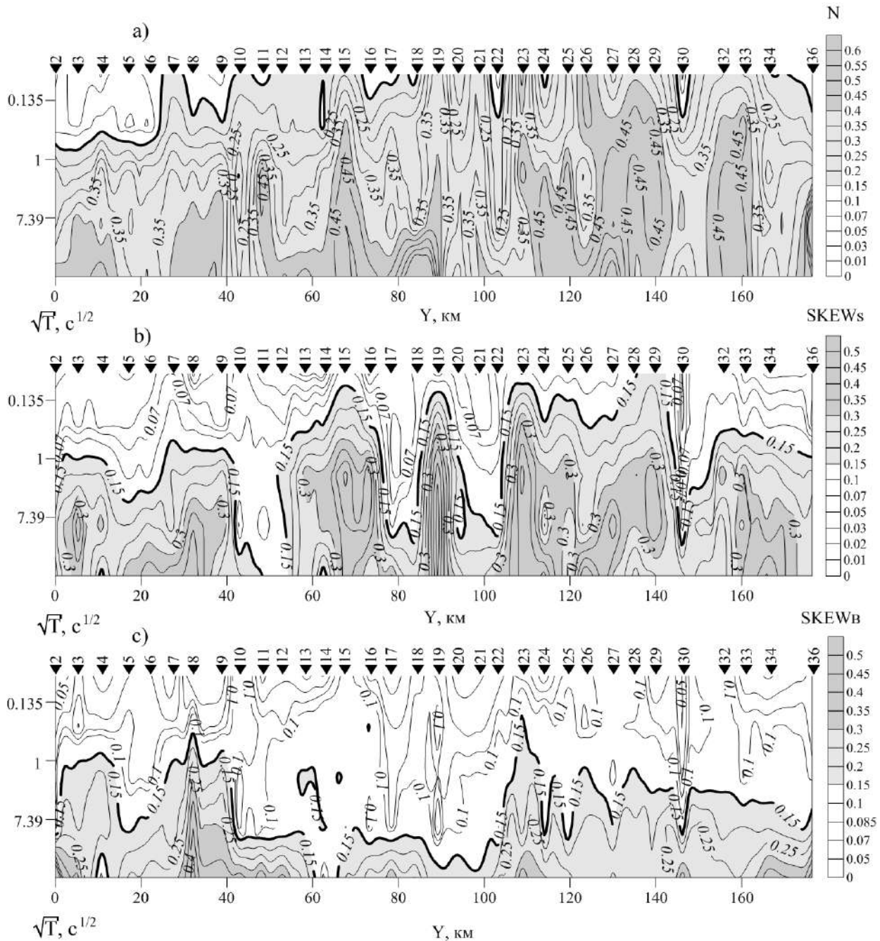
Рис. 2. Частотные разрезы магнитотеллурических параметров:
