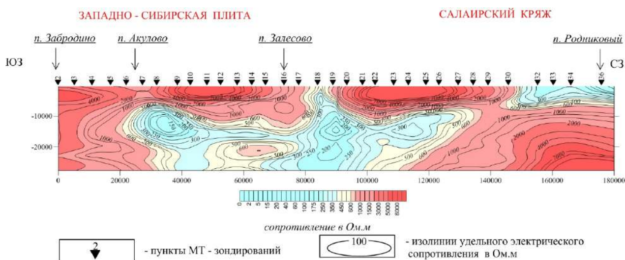
Рис. 3. Глубинный геоэлектрический разрез по профилю п. Тальменка – г. Ленинск-Кузнецкий
